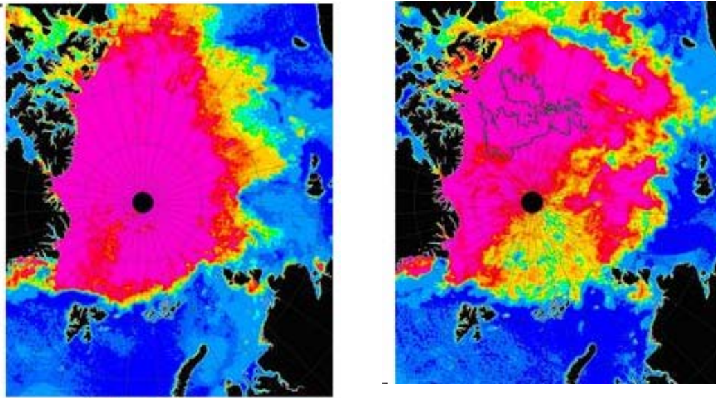
Fig. 1: Les glaces de l'Arctique (en rose) vues par EOS Aqua en août 2005 (à gauche) et août 2006 (à droite)
