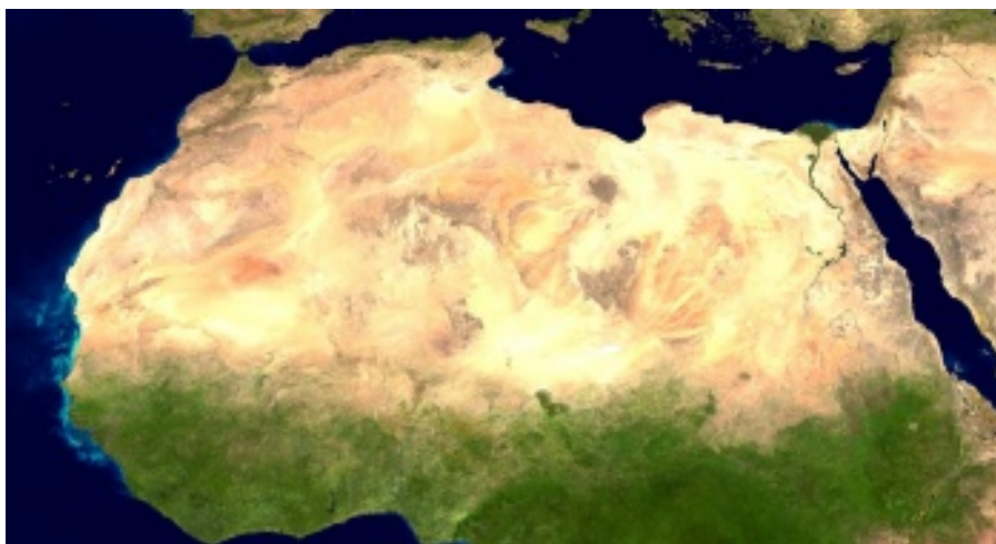
Fig. 2: Image satellite du Sahara africain
